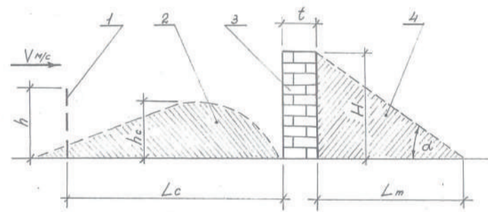
1 – ажурный щит высотой h=1,5-2,0 м с 50...75% проницаемостью; 2 – снежный шлейф, L_c от 50 до 100 м; 3 – ветрозащитная стенка высотой H не более 3 м и толщиной стенок t=1,0-1,5 м из тюков соломы плотностью 120-140 кг/м 3 ; 4 – защитная зона для животных, L_m – длина ветровой тени
