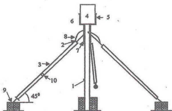
1 – стойка (труба высотой 200 мм, Ø 40 мм); 2 – растяжка из трубы; 3 – тряпичная обвязка; 4 – бачок; 5 – кран; 6 – пружина; 7 – рычаг, Ø 6 мм; 8 – шланг резиновый, Ø 12 мм; 9 – анкерный болт, Ø 25 мм; 10 – смазочные отверстия, Ø 3 мм, Ø 25 мм; 10 – смазочные отверстия, Ø 3 мм.
